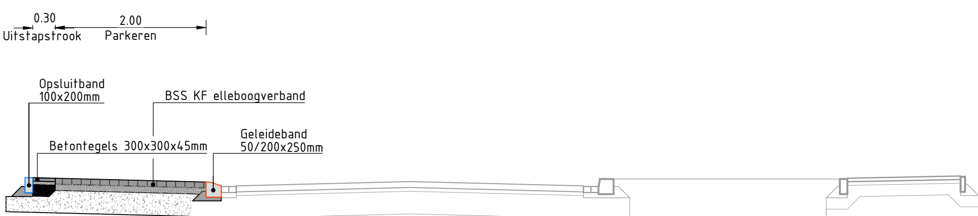
Dwarsprofiel C-C Jan de Oudestraat variant 2 schaal 1:50
