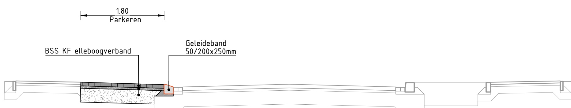
Dwarsprofiel D-D Irenelaan schaal 1:50
